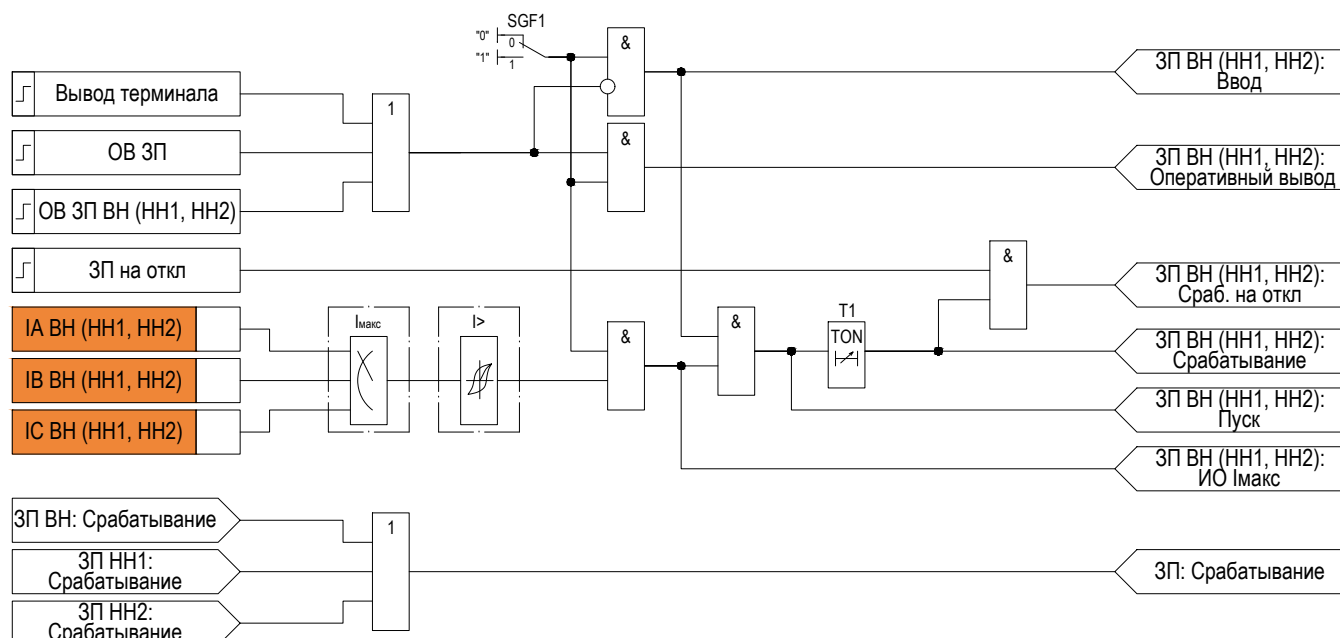
Рисунок 2.14 – Функциональная схема логики ЗП
