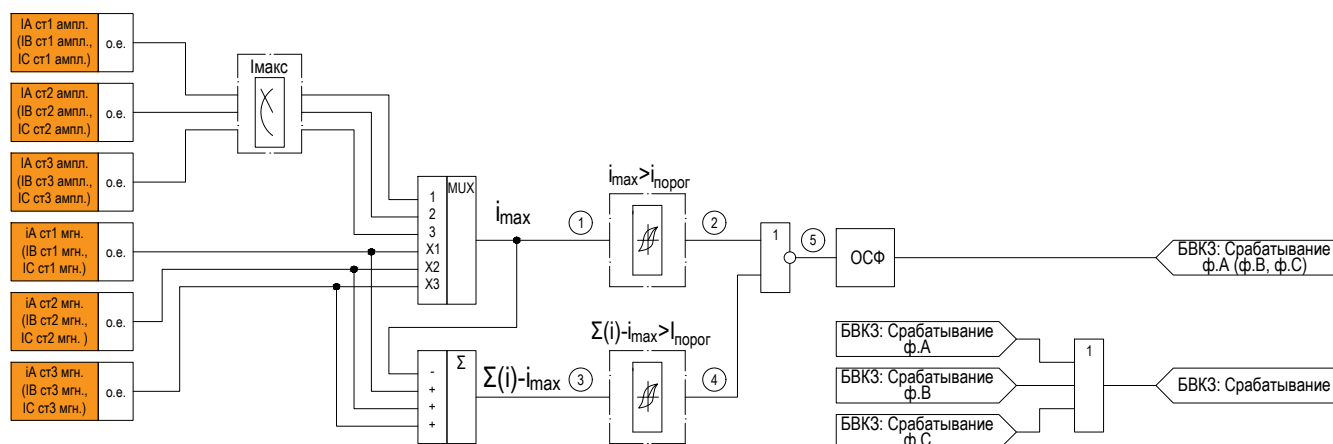
Рисунок 2.8 – Функциональная схема логики БВКЗ
